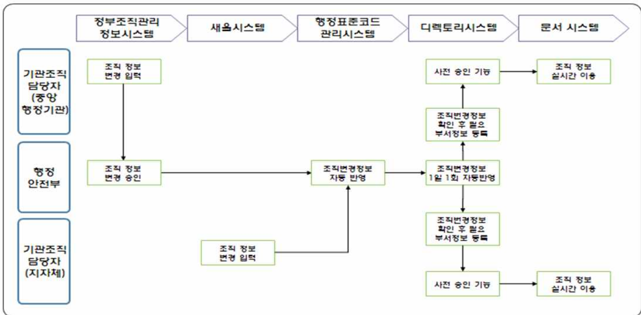
<조직정보 변경 시 반영처리 절차>
