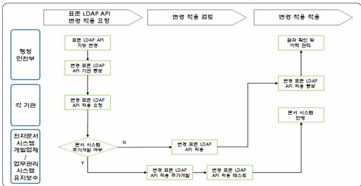
<표준 LDAP API 변경처리 절차>
