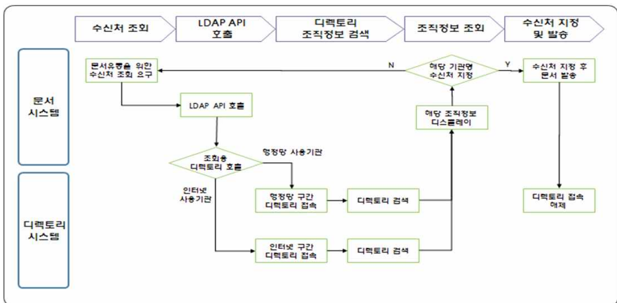
<정부디렉토리시스템의 조직정보 이용처리 절차>
